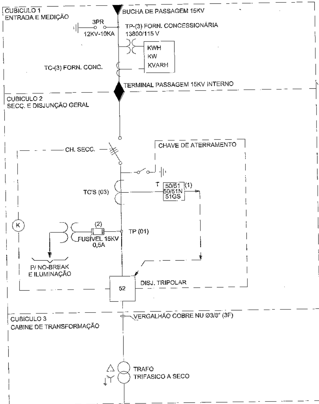
FIGURA 6 – MODELO DE DIAGRAMA UNIFILAR
